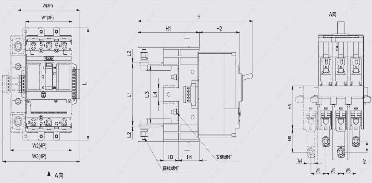
图 15 插入式板后接线（水平）产品的外形尺寸图
