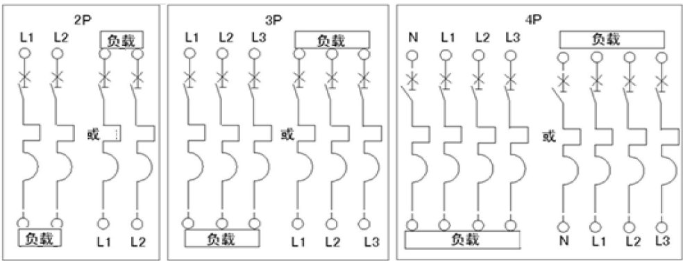
图 5 交流产品接线示意图
