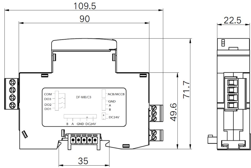
图 30 通信适配器外形尺寸图
