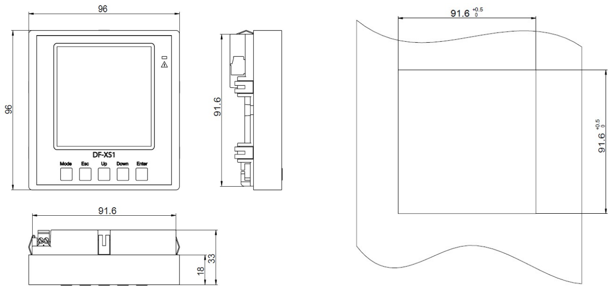
图 33 显示模块外形尺寸图
