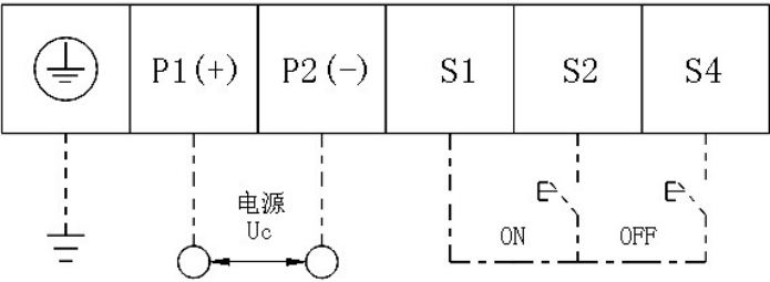
图 21 电操接线图
