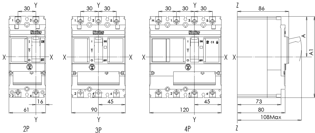
图 7 板前接线产品外形尺寸图
