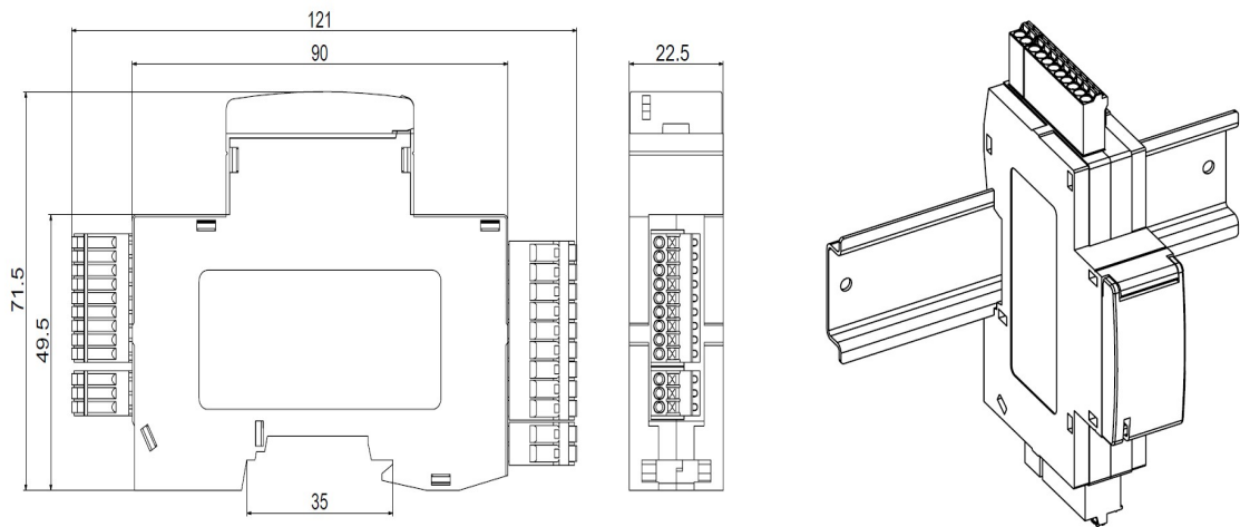
图 35 温度模块外形尺寸图
