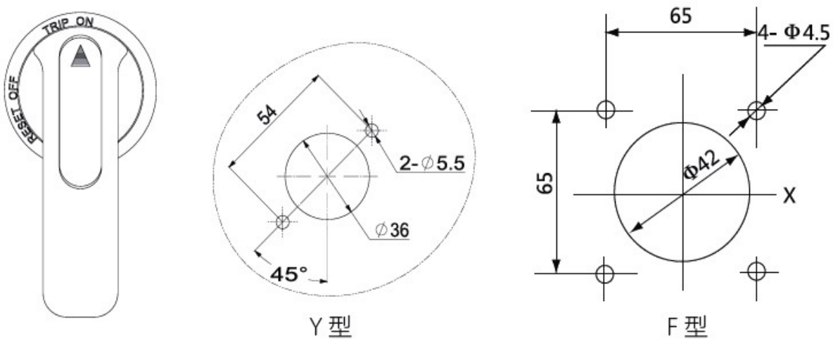
图 23 手动操作手柄开孔尺寸图
