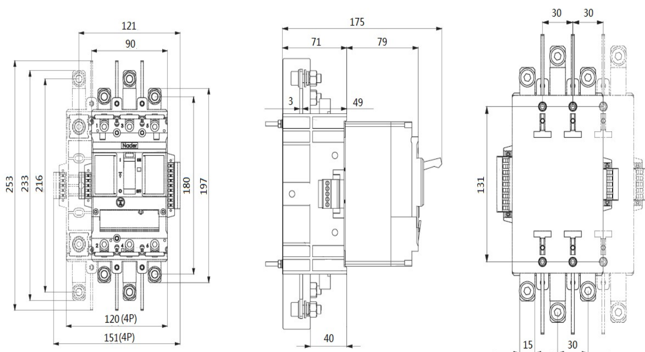
图 13 插入式板前水平接线外形尺寸图
