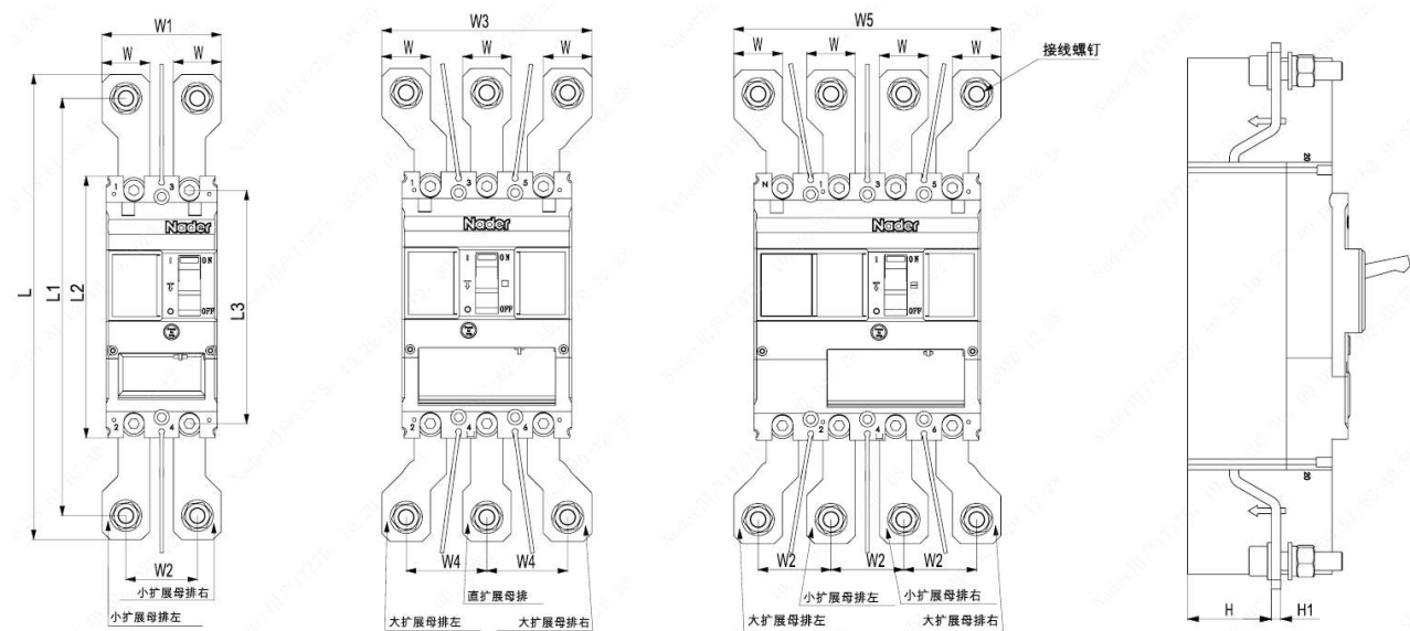
图 8 板前加长扩展接线外形尺寸图
