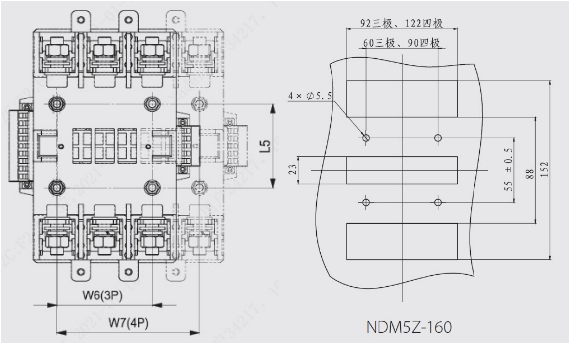
图 16 插入式插座安装板开孔尺寸图
