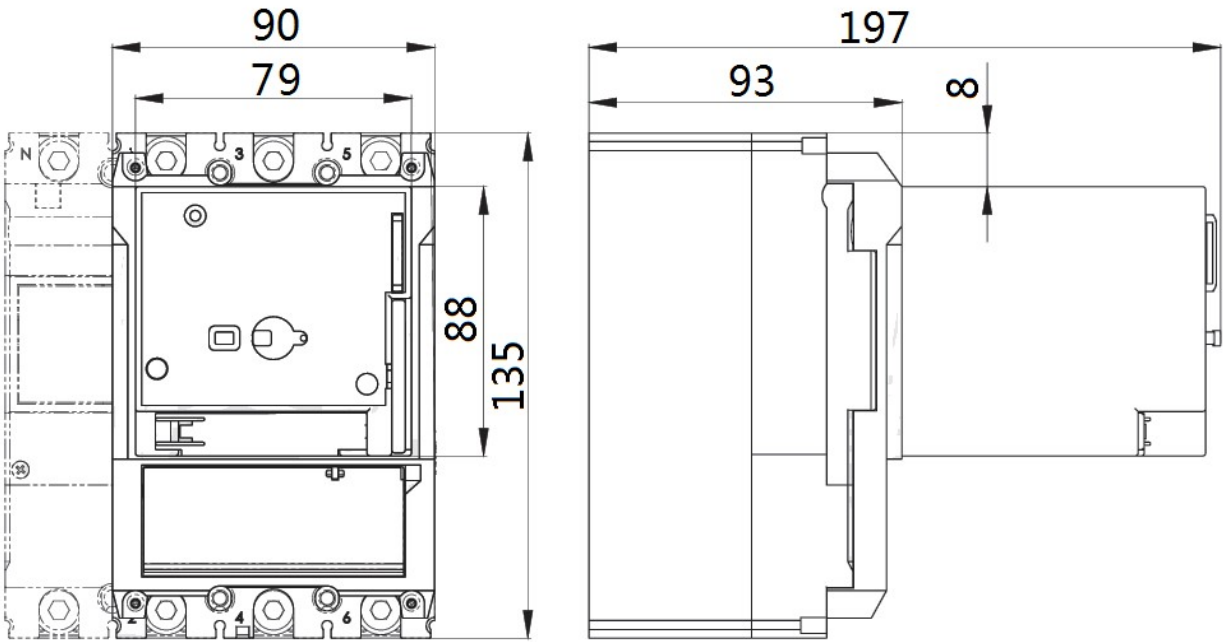
图 20 电动操作外形尺寸图
