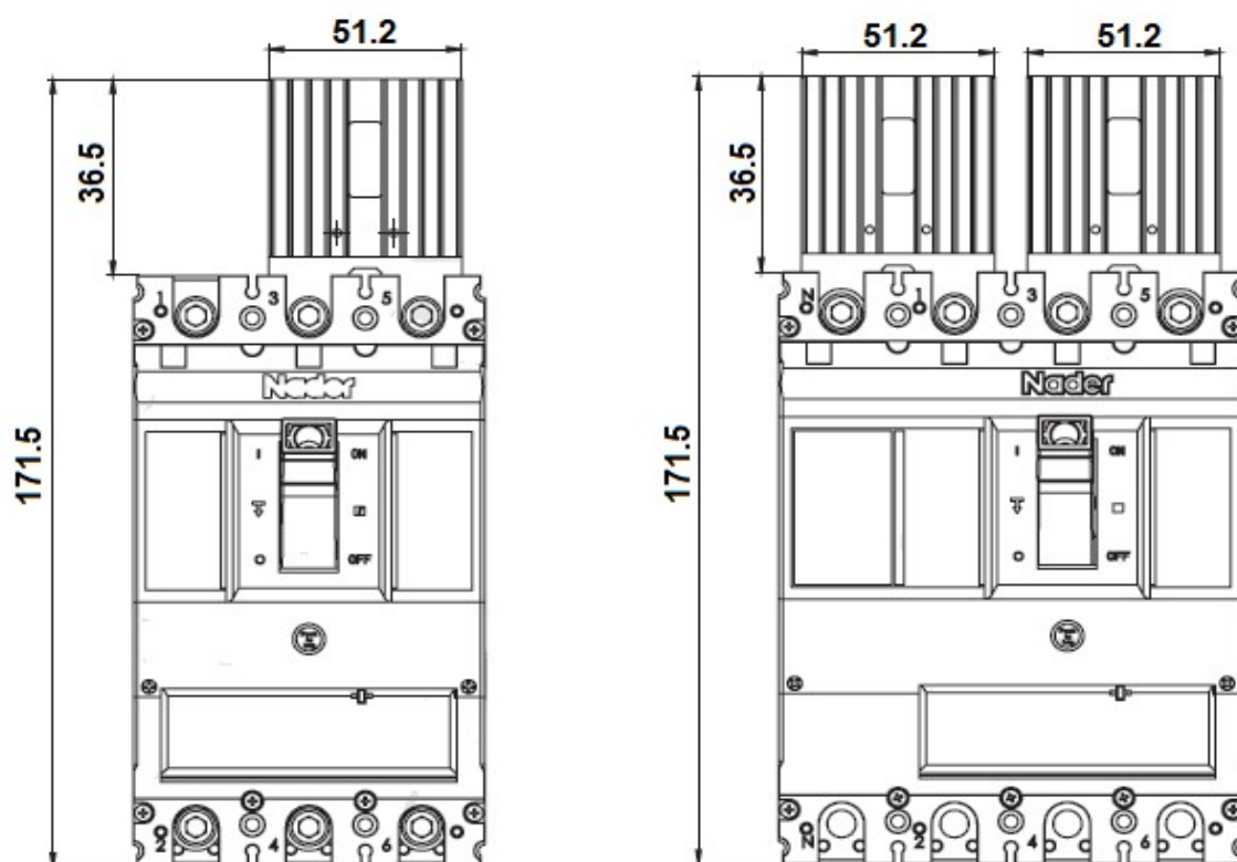
图 11 增加散热附件的产品外形尺寸图
