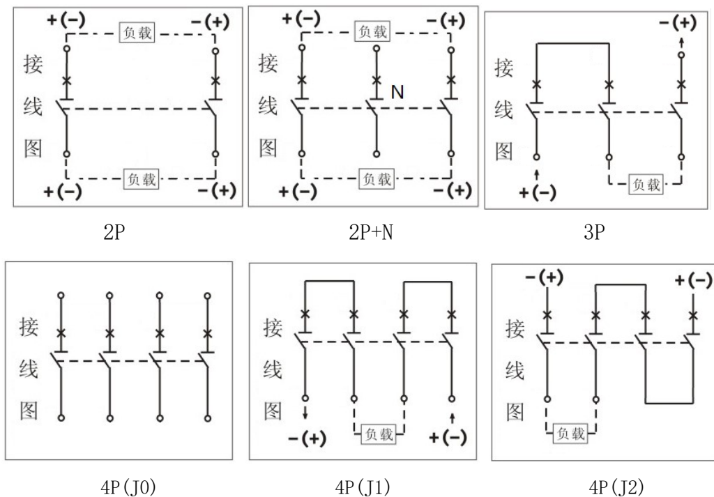
图 6 直流产品接线示意图
