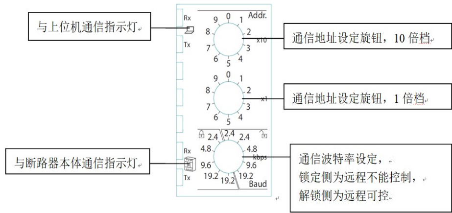
图 31 通信适配器调节档位图
