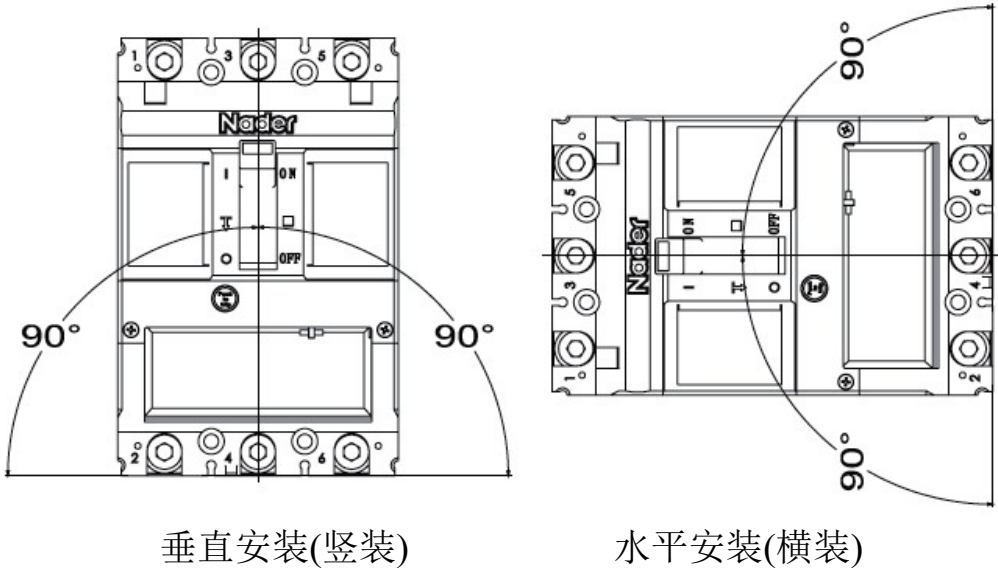
图 26 产品安装方式示意图
