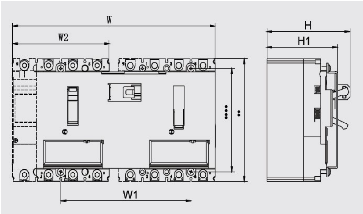
图 18 机械连锁机构与断路器安装后的外形尺寸图
