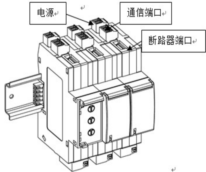
图 32 通信适配器端口示意图
