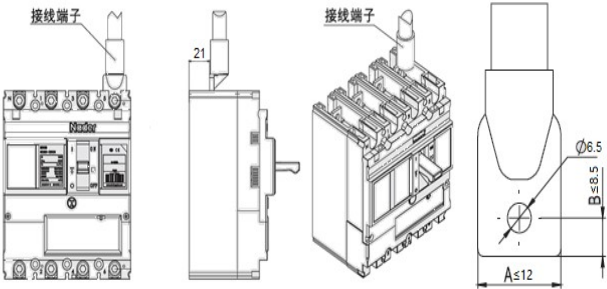
图 24 板前铜排或带接线端子的铜电缆连接图
