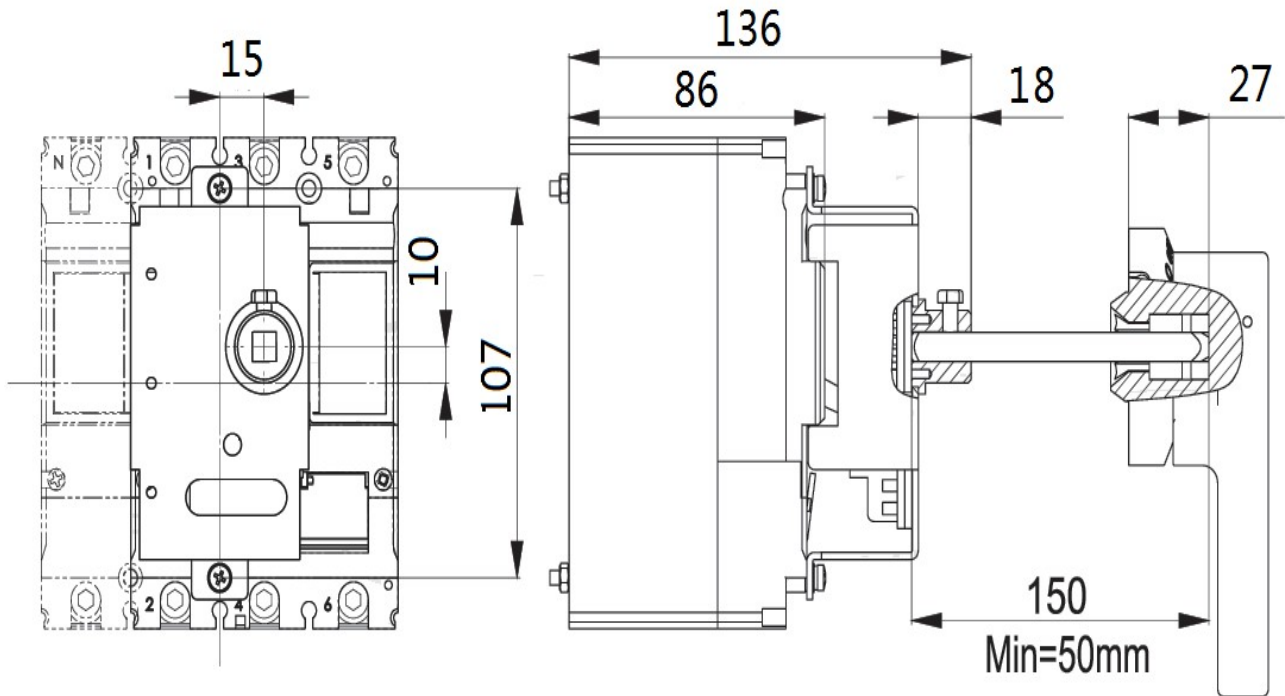
图 22 手动操作外形尺寸图
