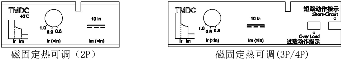
图 4 直流保护调节档位图
