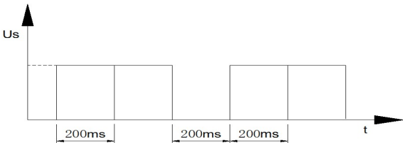
图 29 分励脱扣器工作原理图
