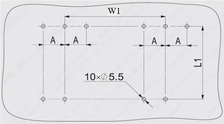
图 19 安装开孔尺寸图
