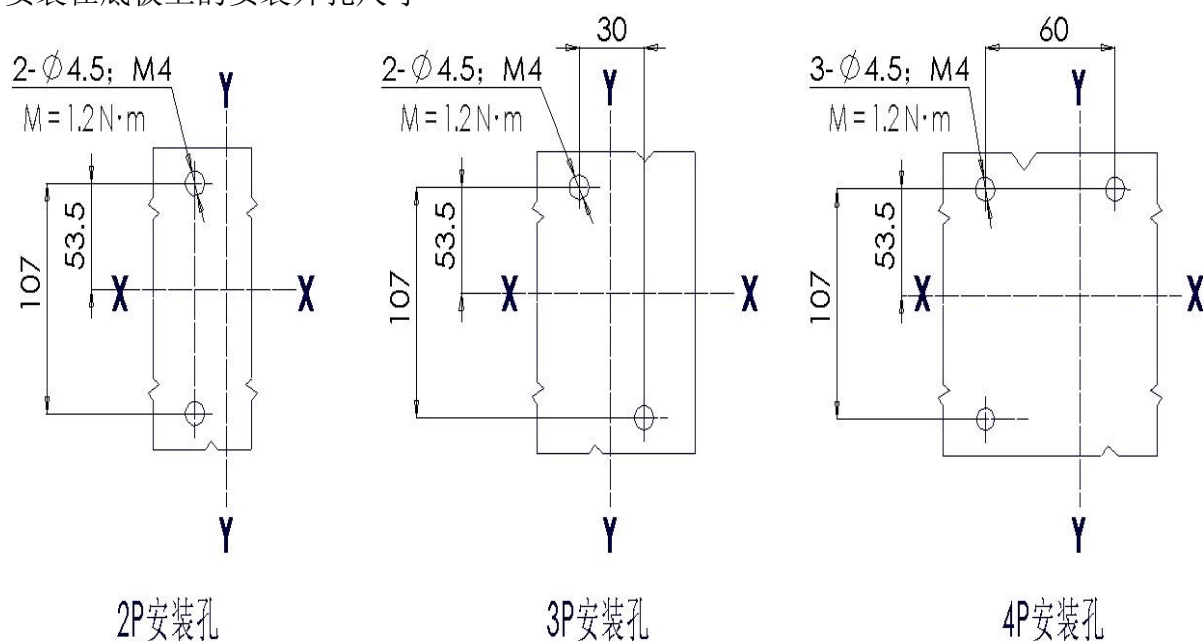
图 12 安装开孔尺寸图
