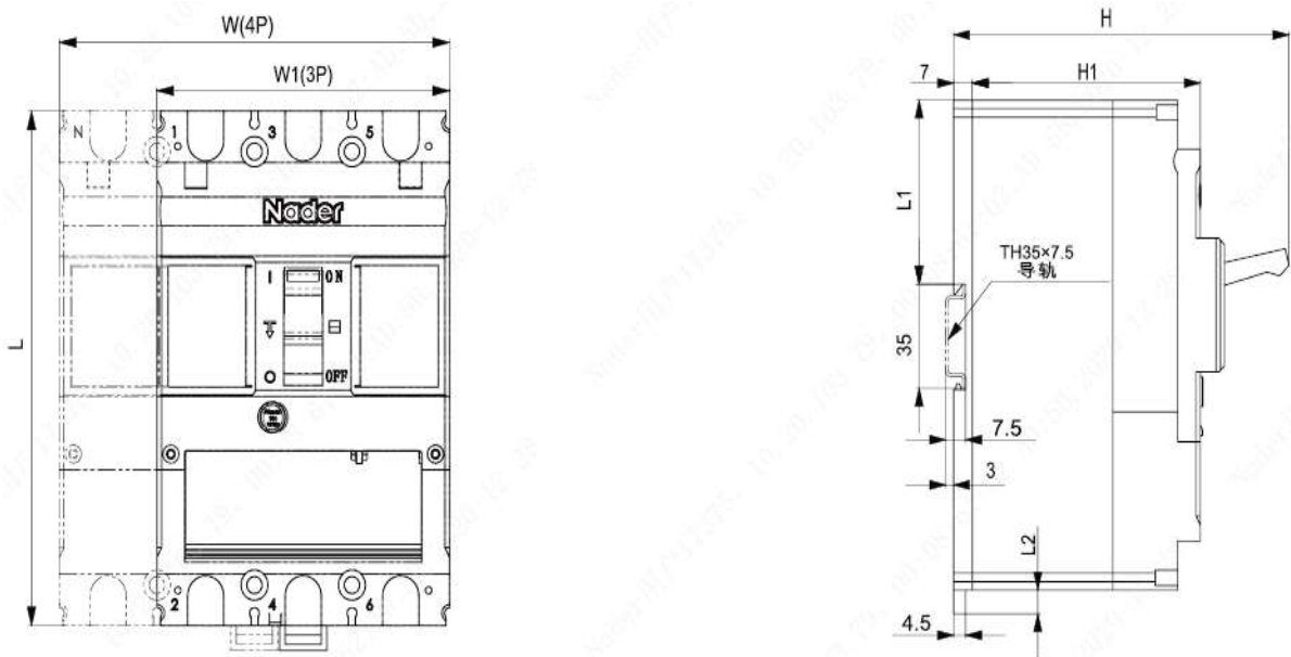
图 17 导轨安装外形尺寸图
