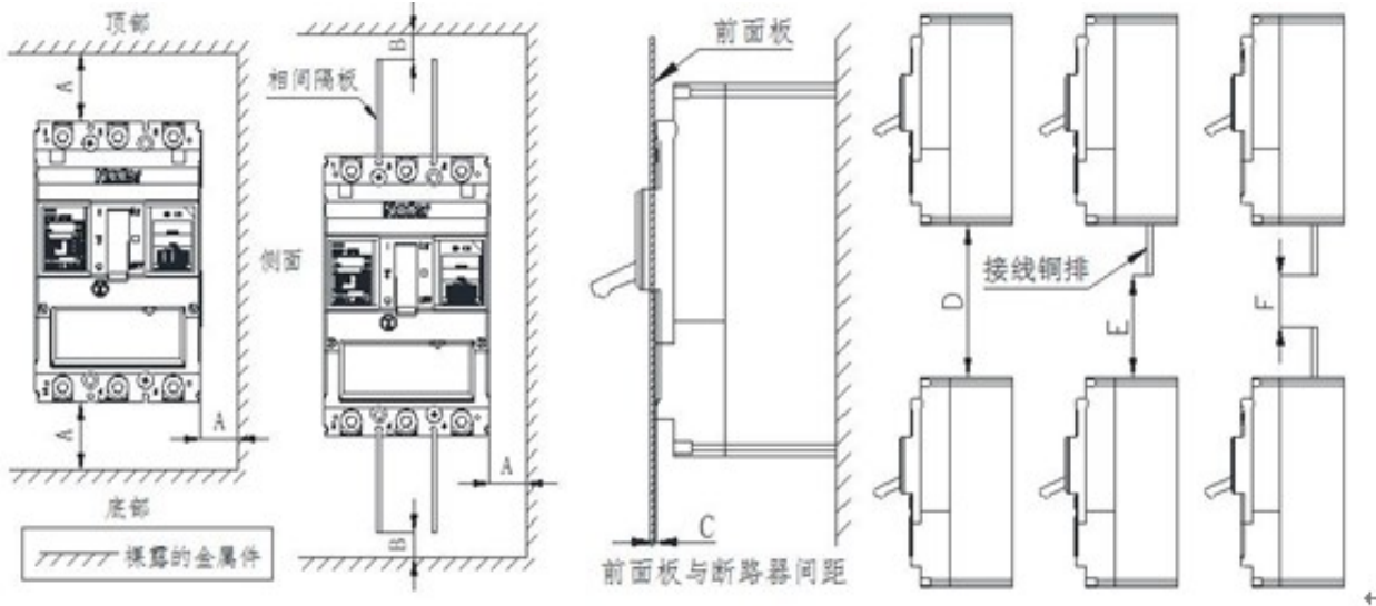
图 25 安全距离示意图
