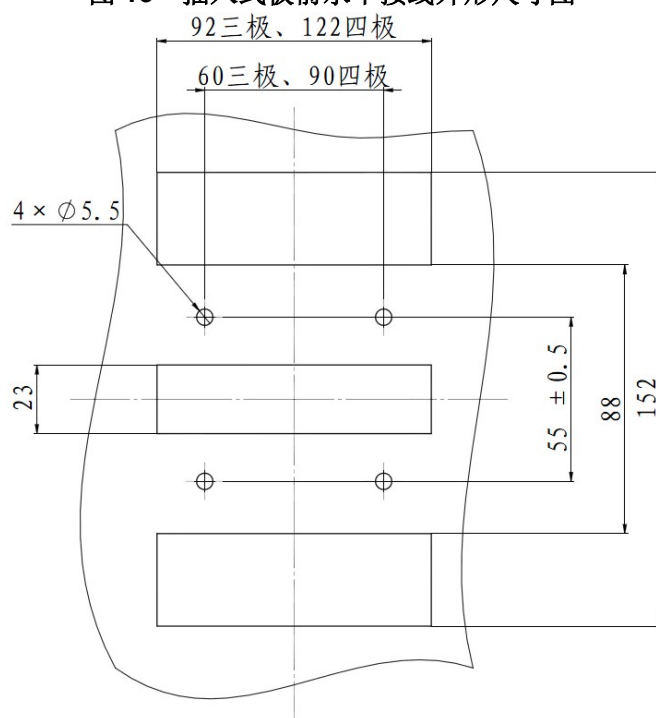
图 14 插入式开孔尺寸图
